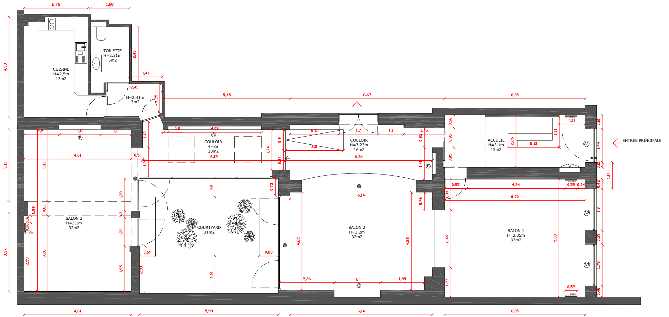
PLAN D'ÉTAGE 0m 1m 2m
