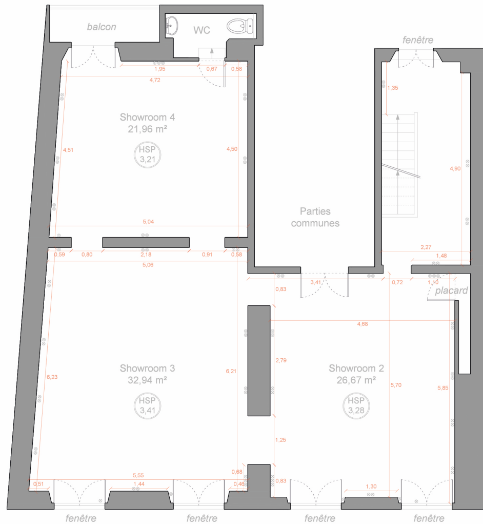
PLAN 1ER ÉTAGE
