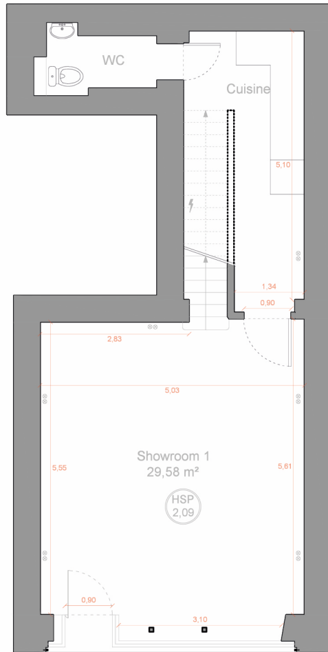
PLAN REZ-DE-CHAUSSÉE
